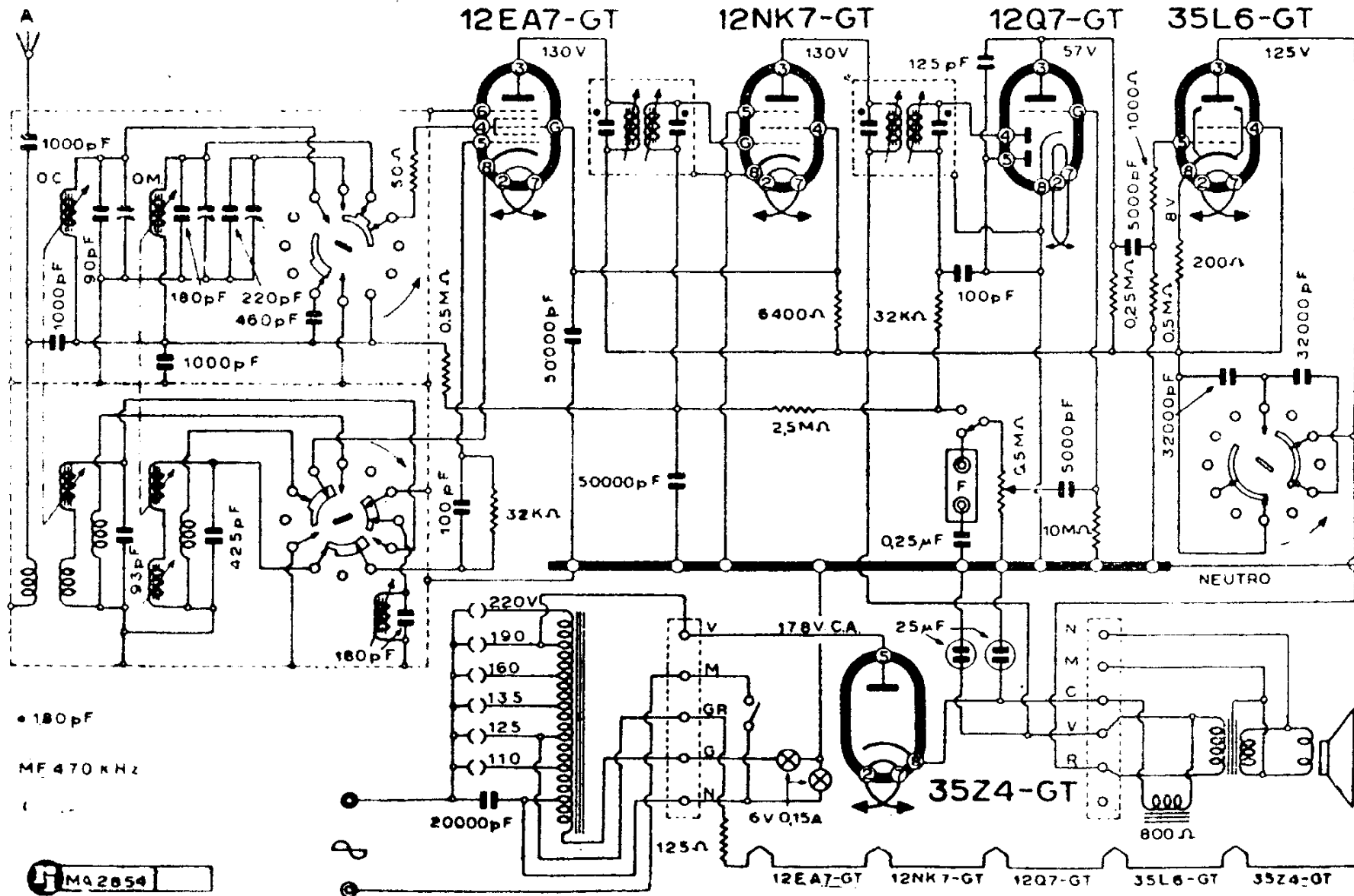
RADIOMARELLI - MOD. « 9A75 »
